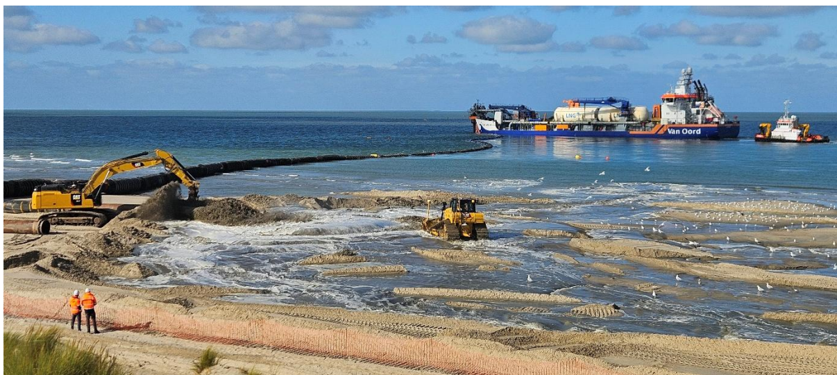
Figuur 1: Vox Apolonia aan het walpersen. Werkschip Panda heeft de Vox Apolonia verbonden met de leiding.
