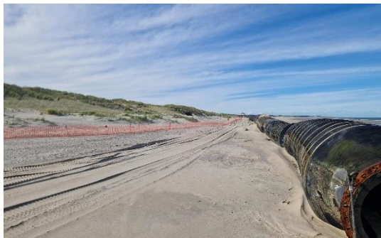
Figuur 1: Drijvende leiding installatie
